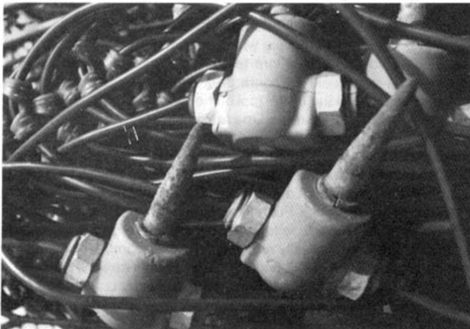
Geophones.
